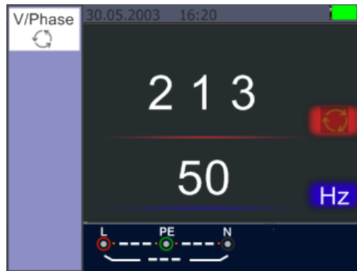
Pantalla de secuencia de fase cuando se conecta en sentido antihorario
