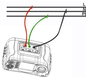
Impedancia de línea L-N (conexión de sondas de test)
